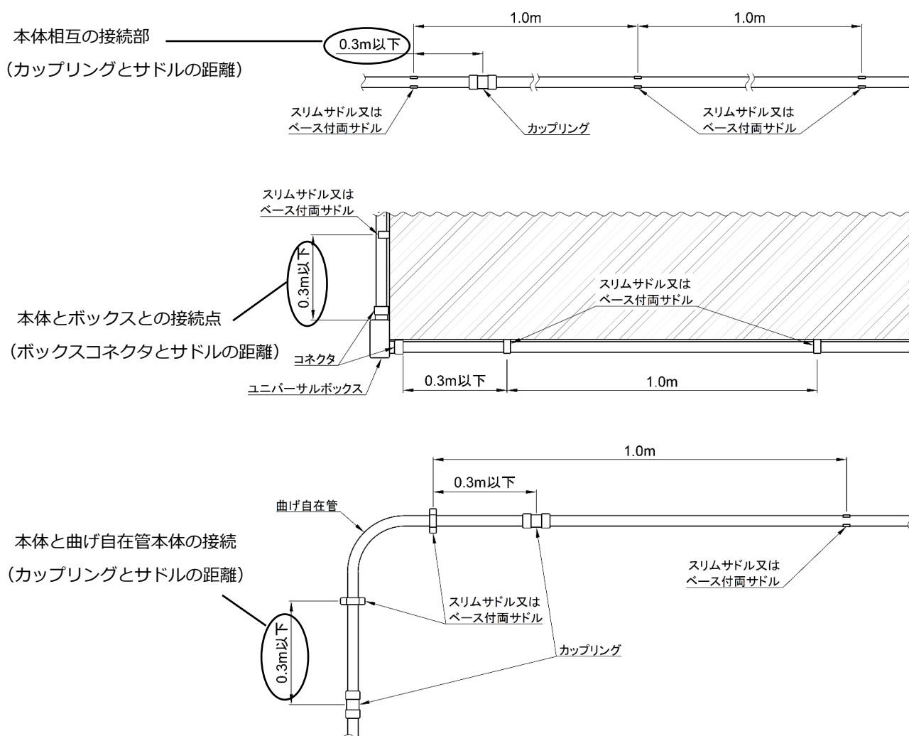
配管例
