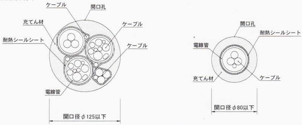
正面図
