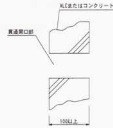
<側断面図>
