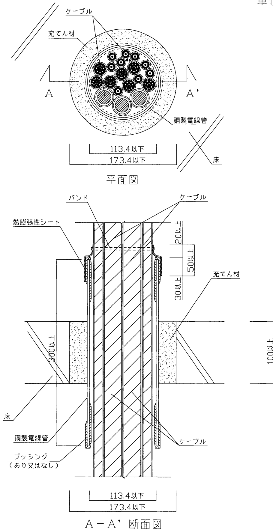
図1 構造説明図
