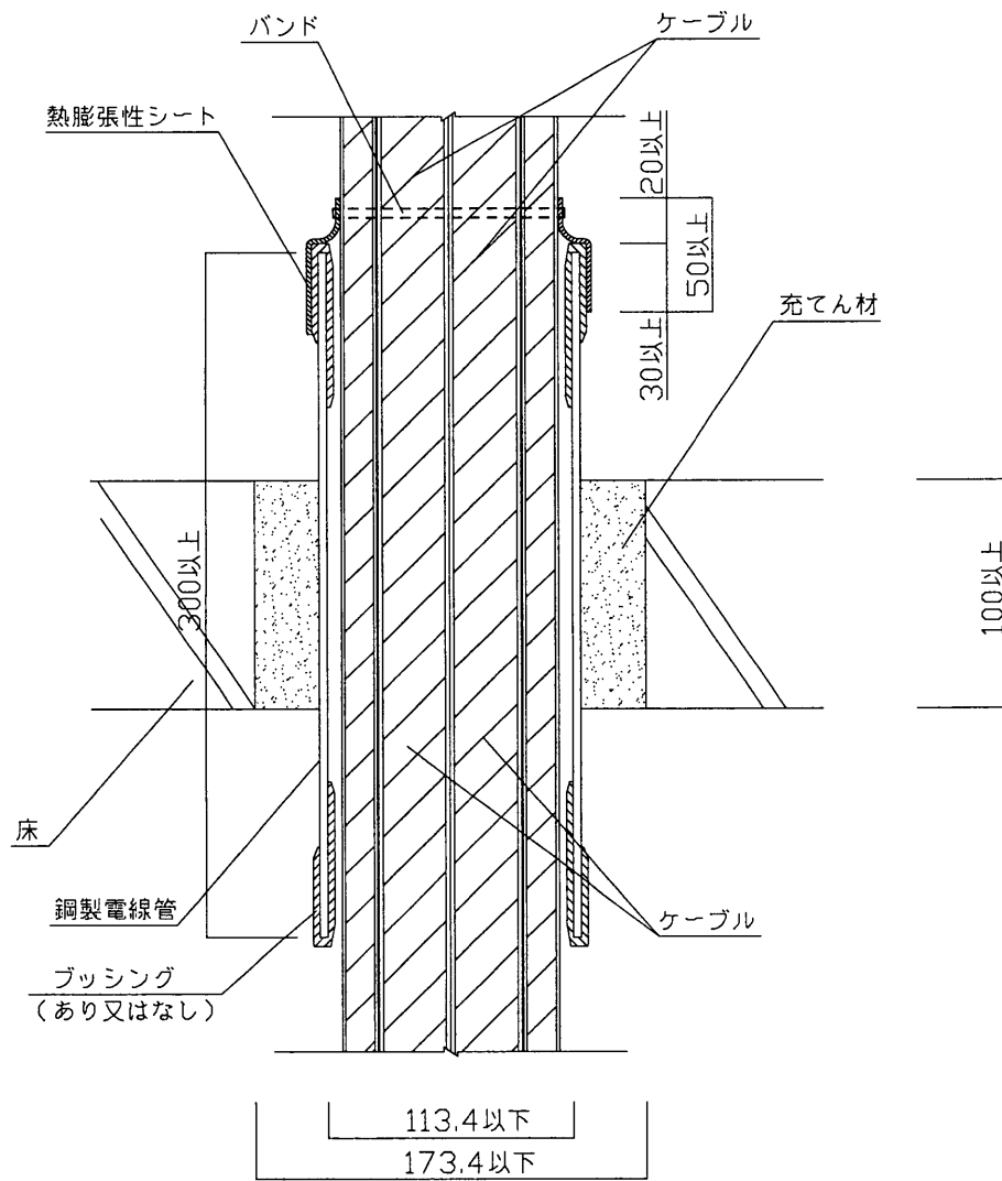
A - A' 断面図
