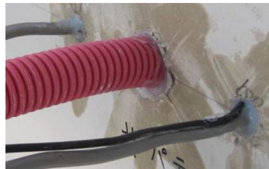
写真-6 ケーブル側状況 (非加熱側)
