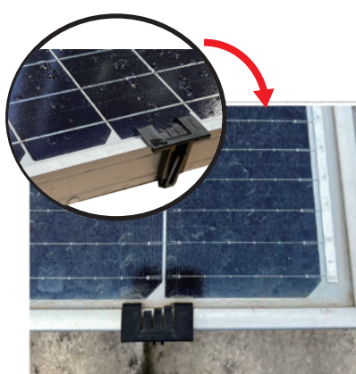
ドレインクリップを装着することで、 排水され、汚れにくくなります。
