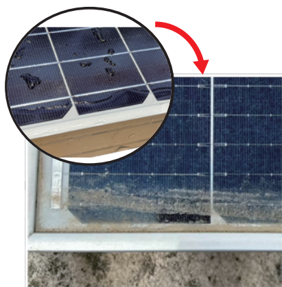
ドレインクリップ未装着時は水が溜まり、 ホコリやコケが付着しやすくなります。
