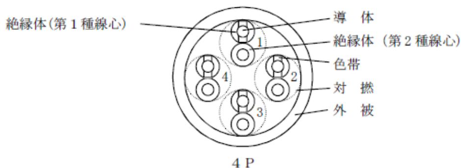
構 造 図
