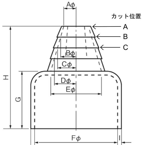
トリプレックス専用 引込管防水ゴムカバー
