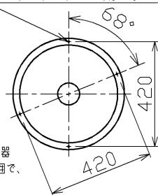
取付けピッチ寸法図 4-φ4.5木ねじ用K.〇
