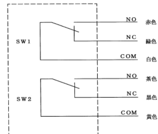
結線図
