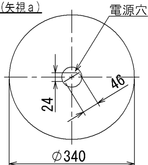
取付寸法(矢視a)
