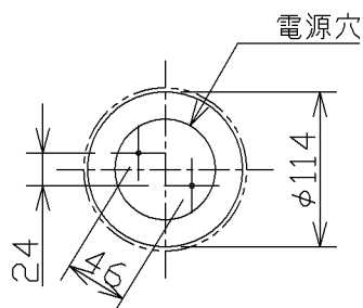
取付寸法（矢視②）
