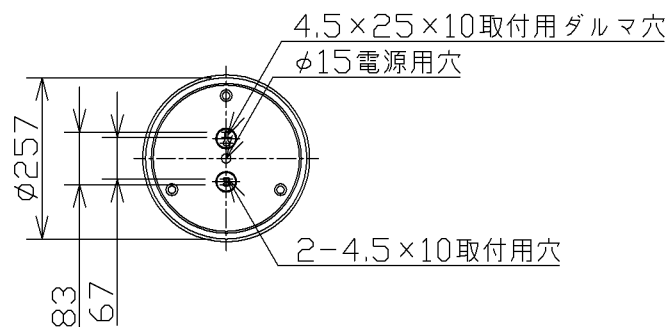
取付寸法（矢視②）
