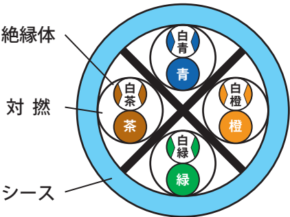
構造図
