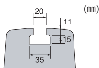
断面図
