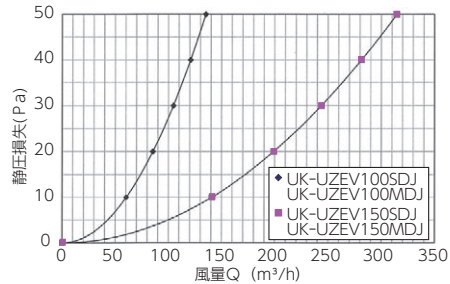
■ 静圧損失特性(防火ダンパー付)
