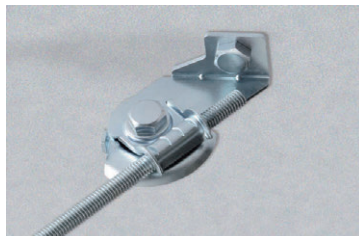
▲FL-E-JP クロスロック®Eタイプ(ボルト固定式)
