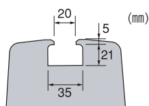
断面図
