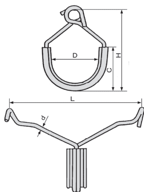
受具断面図
