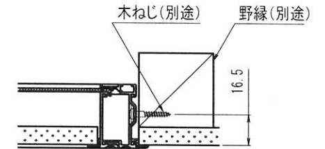
木製天井地下断面納まり図
