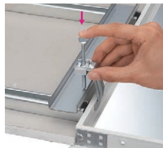
②ハンガーボルトを取付野縁に当たるところまで押し込む
