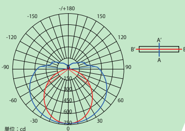
■配光図
