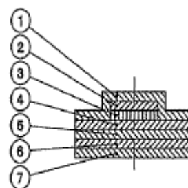
基本積層構造図
