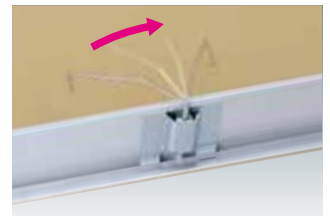
天井仕上材の厚み(3~28mm)に関係なく、ばね材を回転させるだけで内枠ボード材の素早い固定が可能
