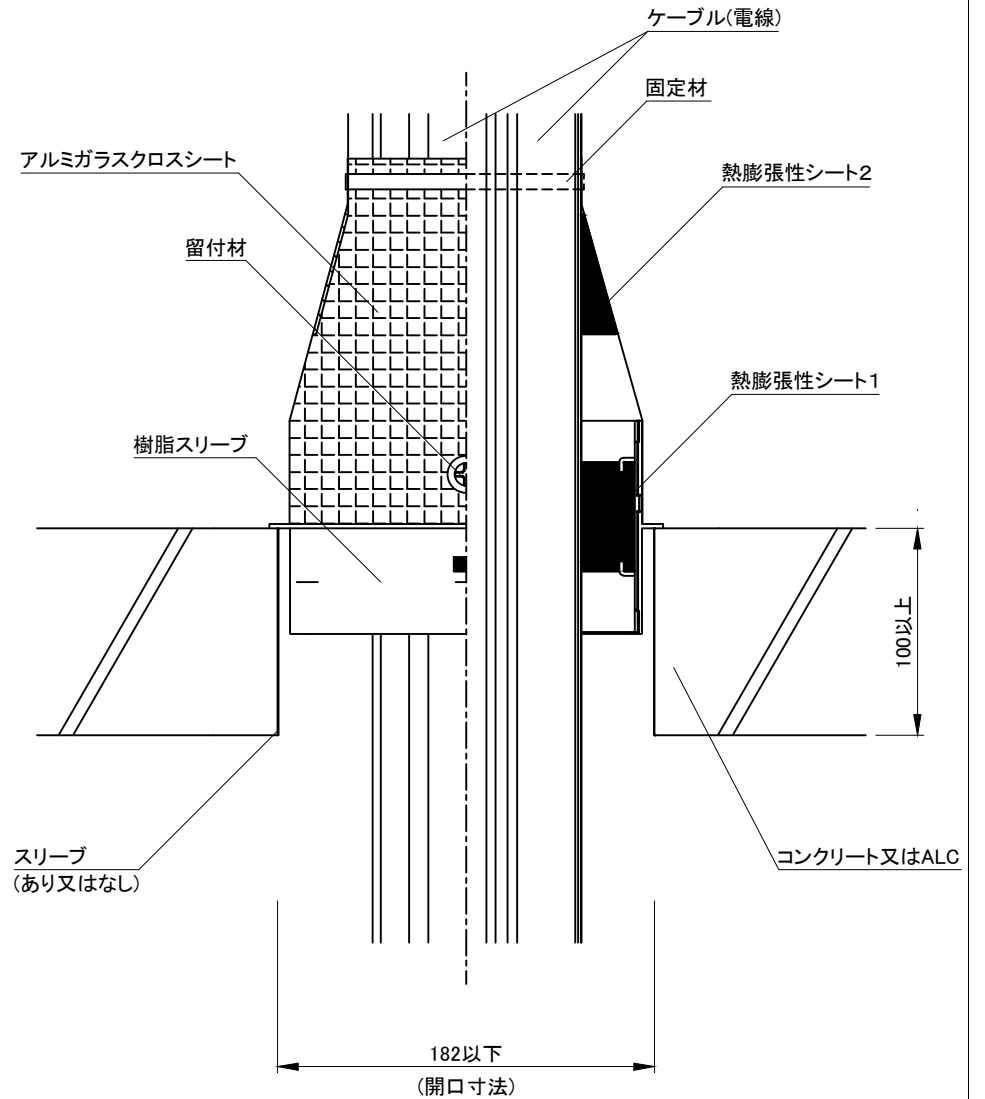
断面図
