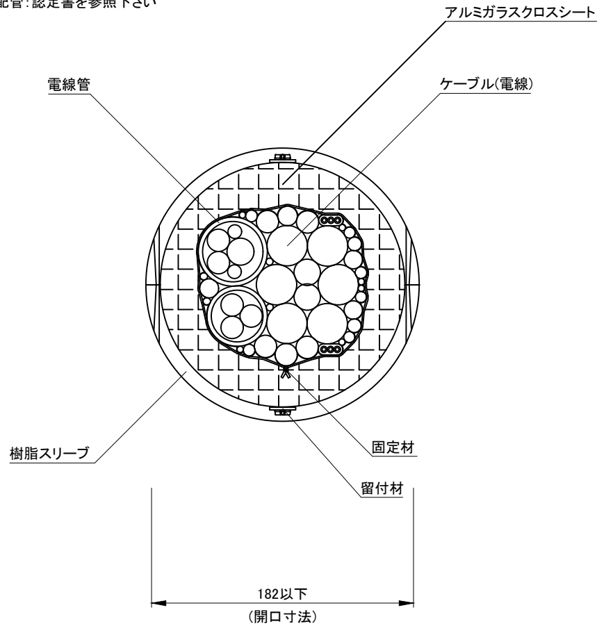
平面図
