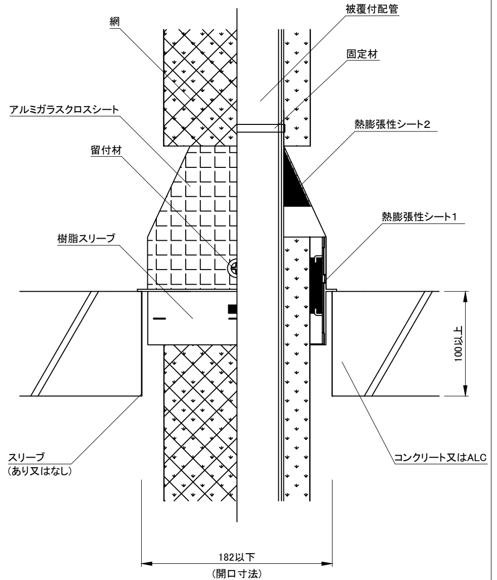
断面図
