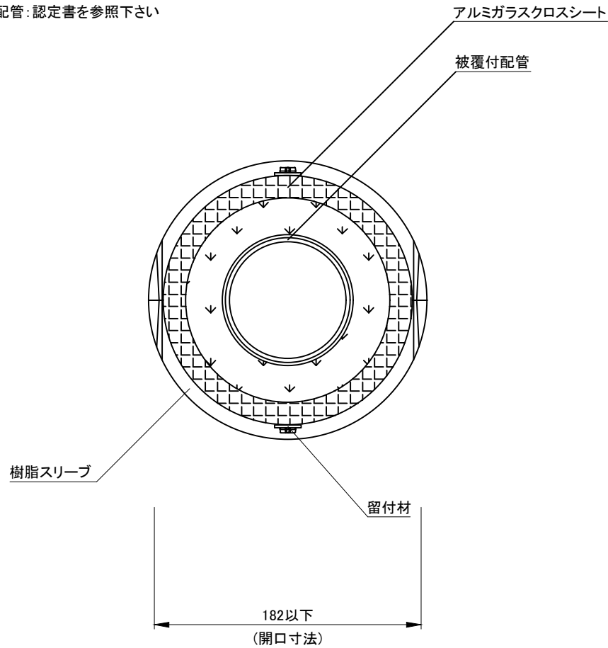
平面図
