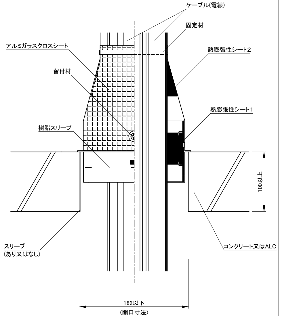
断面図
