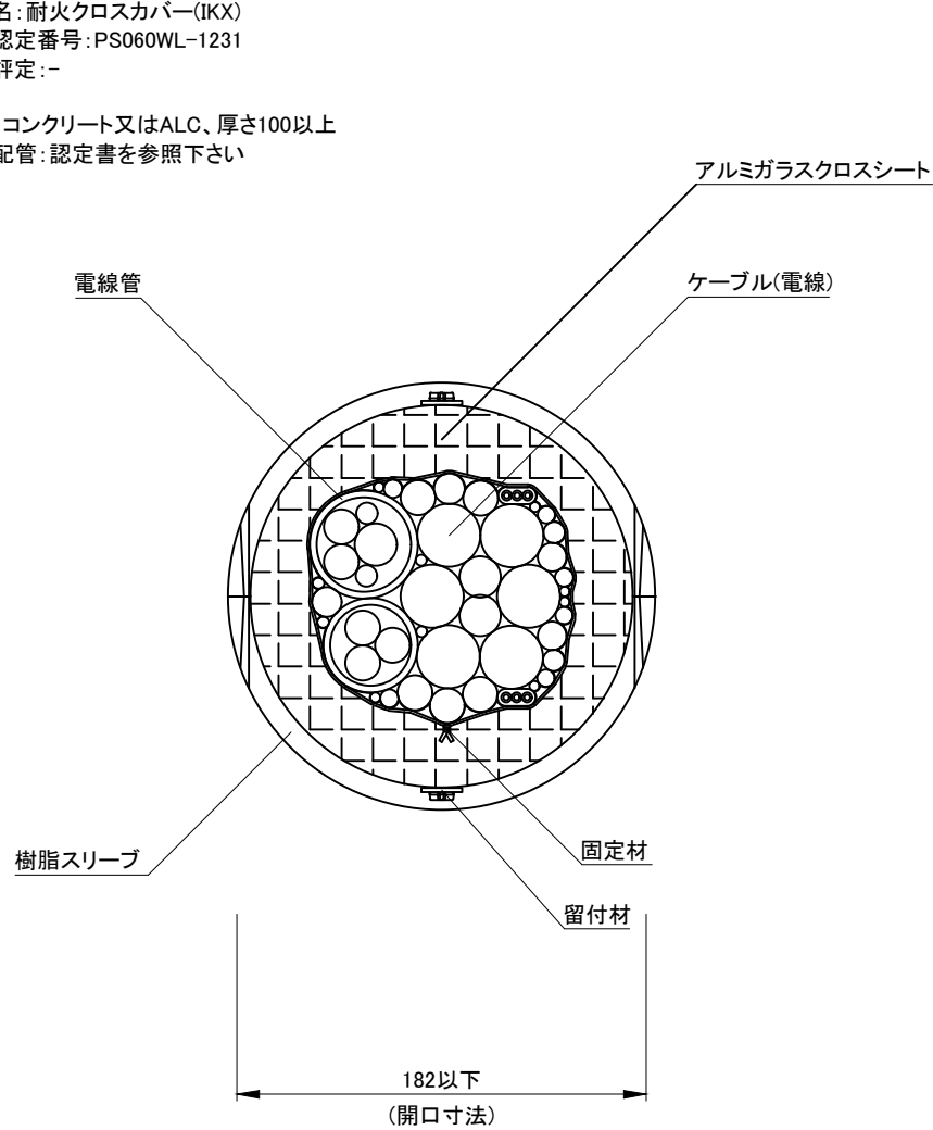
平面図
