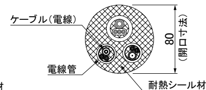
背面図
