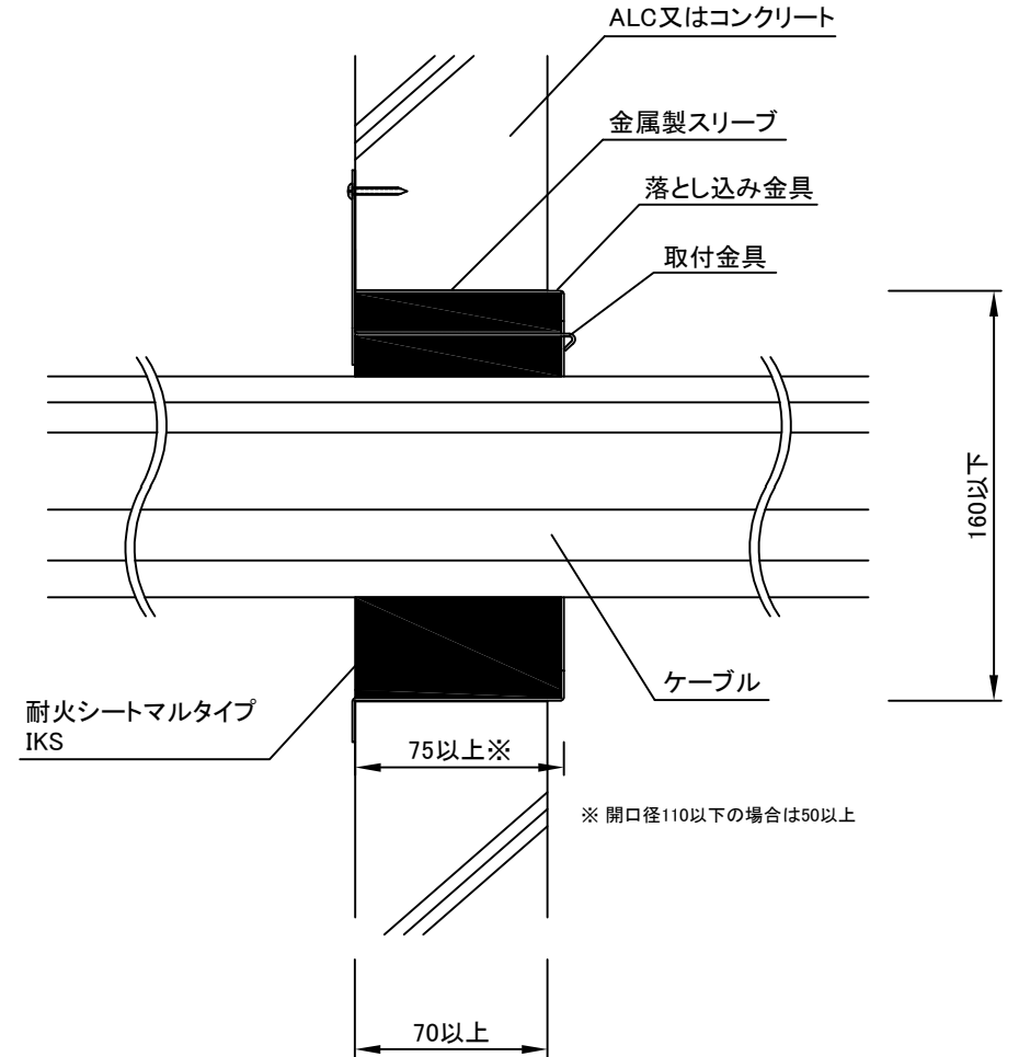
断面図
