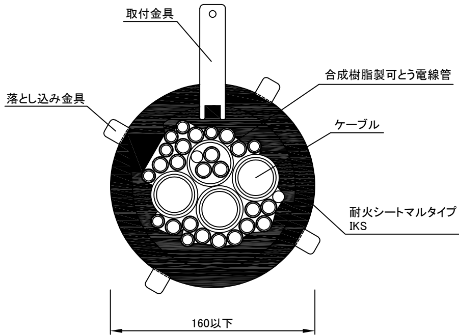
正面図
