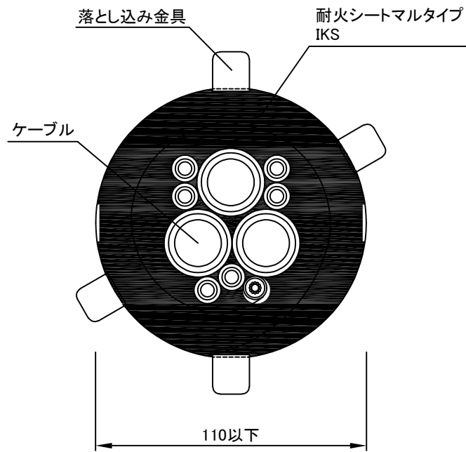
正面図
