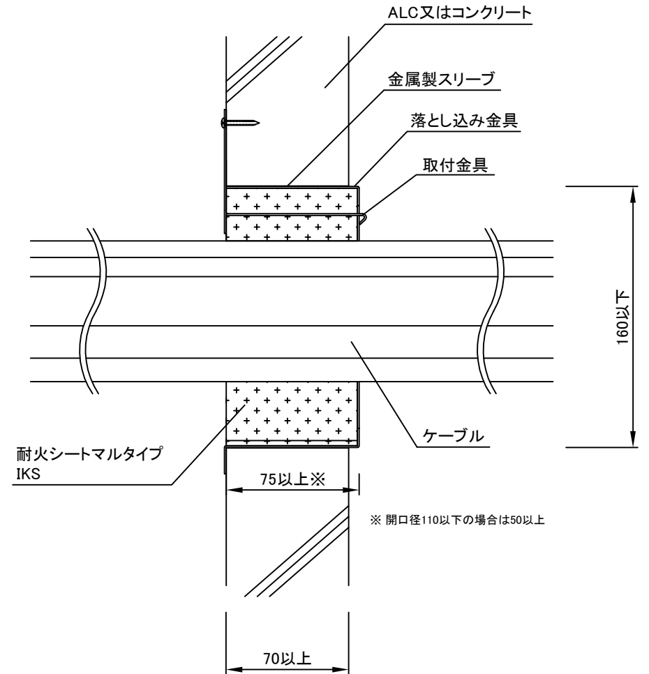
断面図
