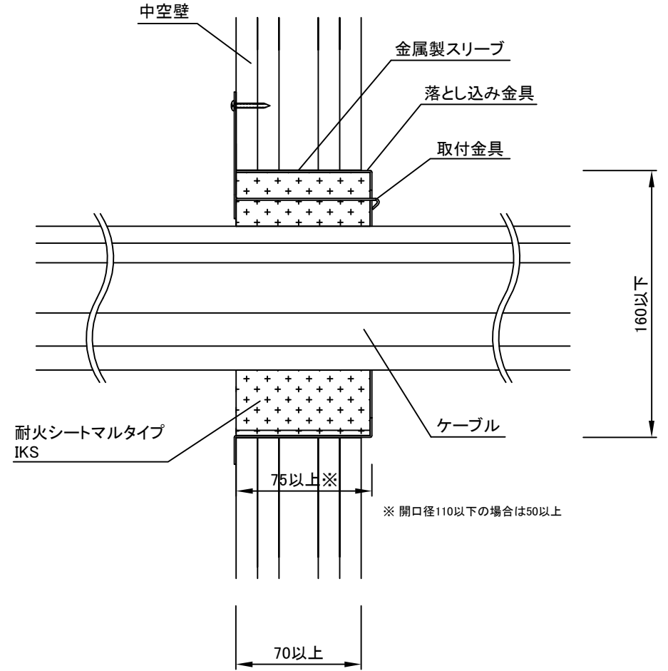
断面図
