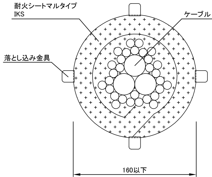
平面図
