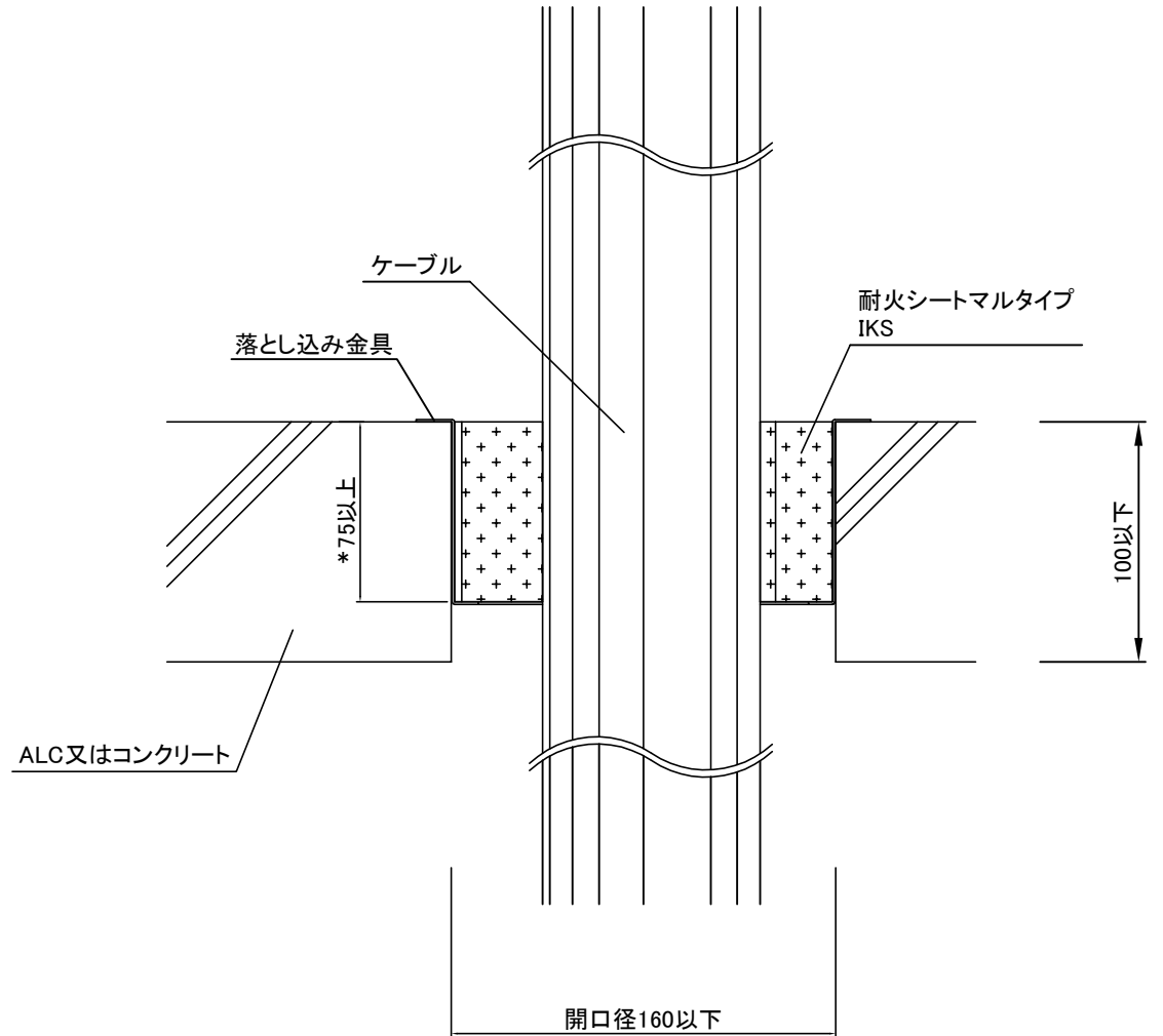
断面図
