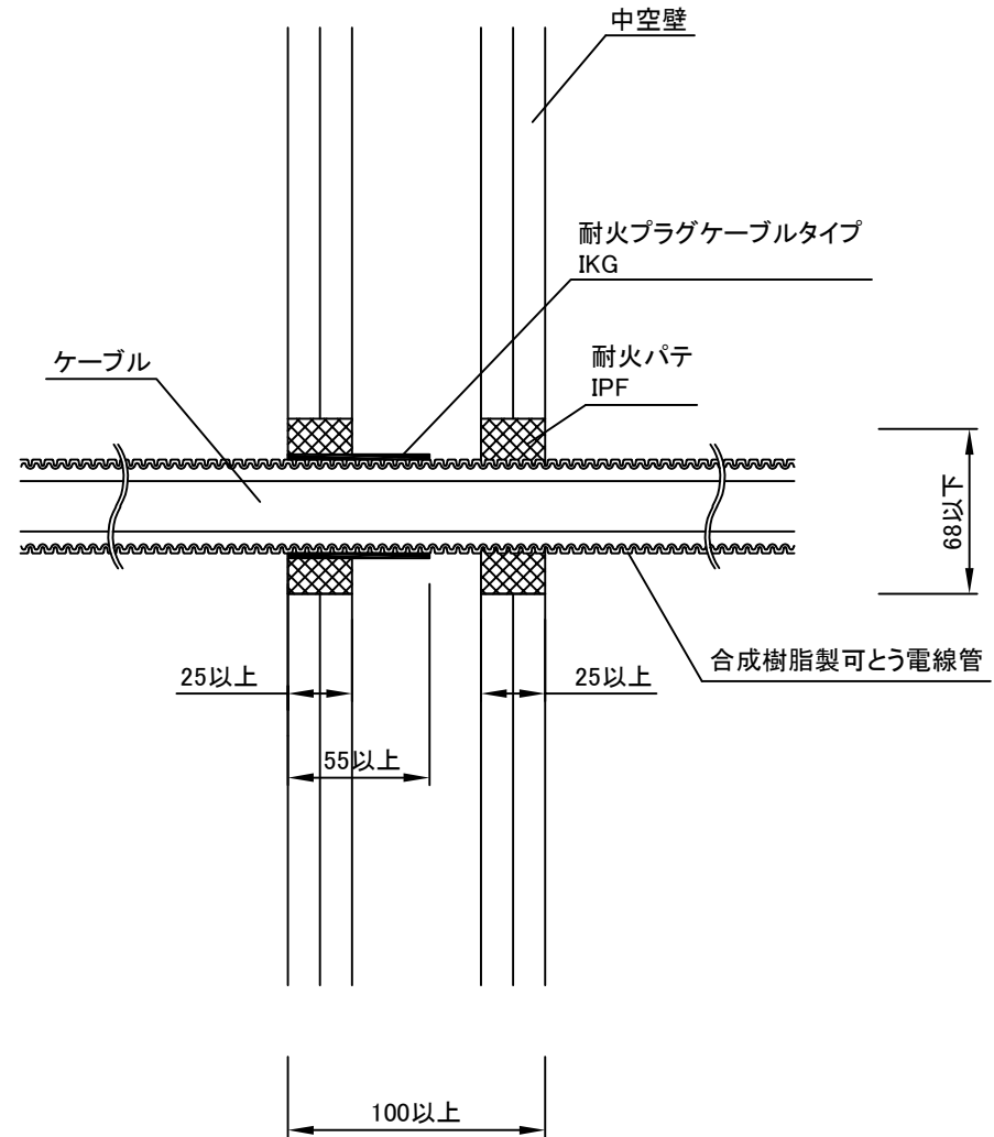
断面図
