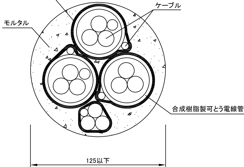
正面図
