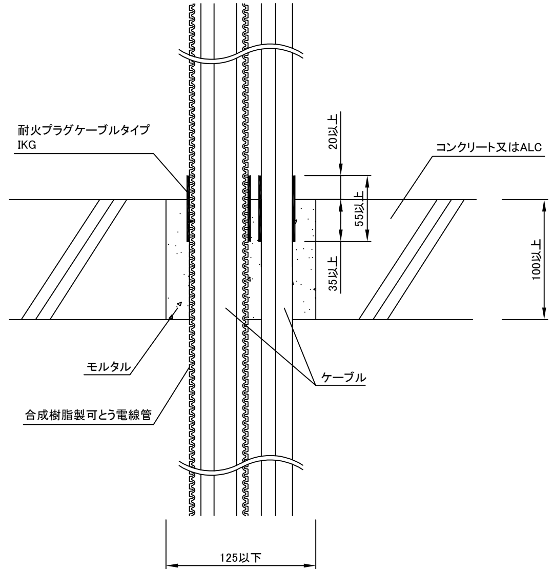
断面図
