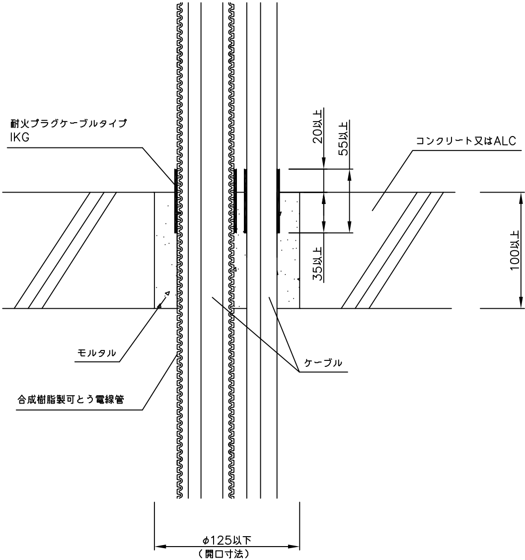
断面図
