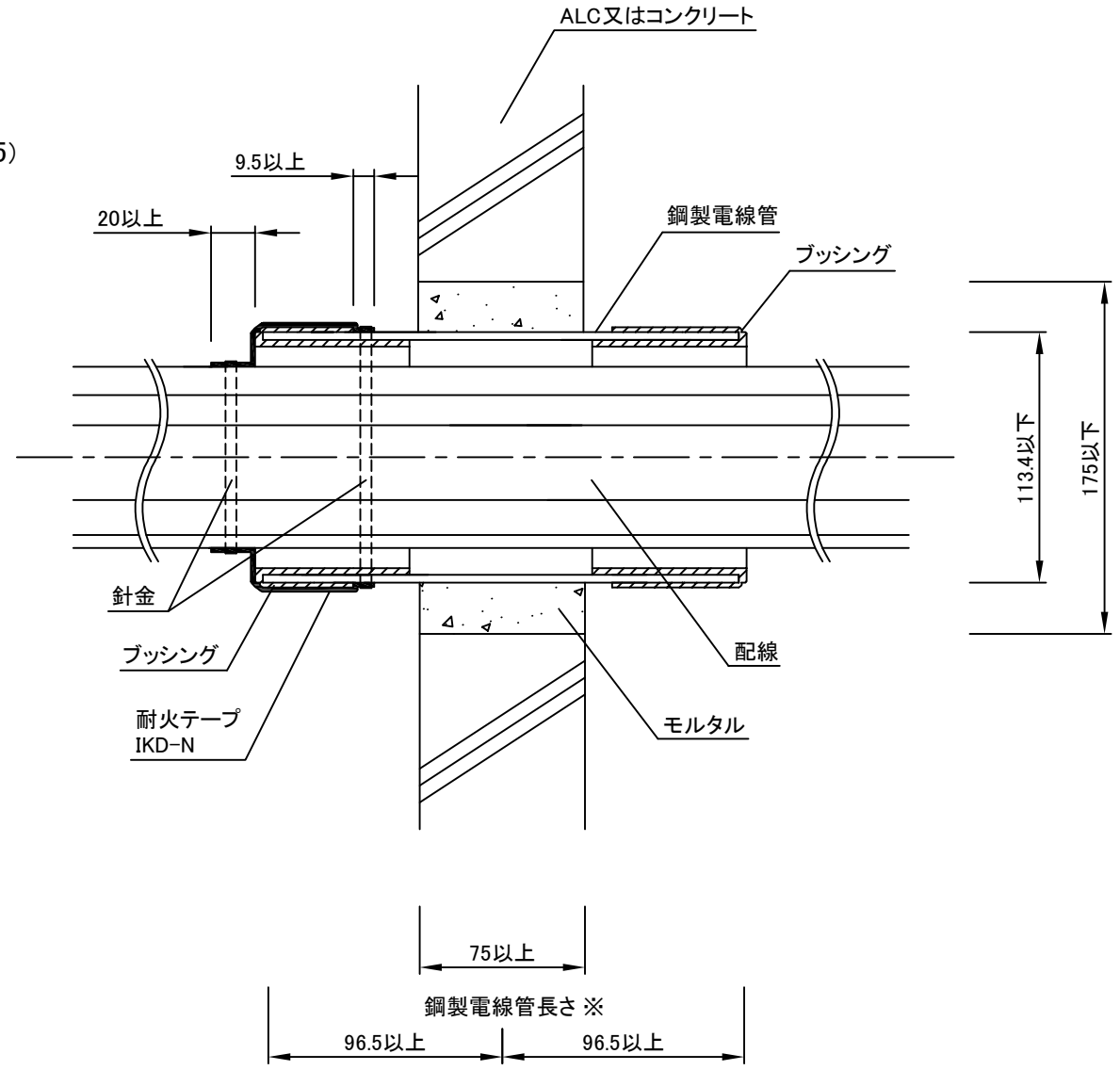
断面図
