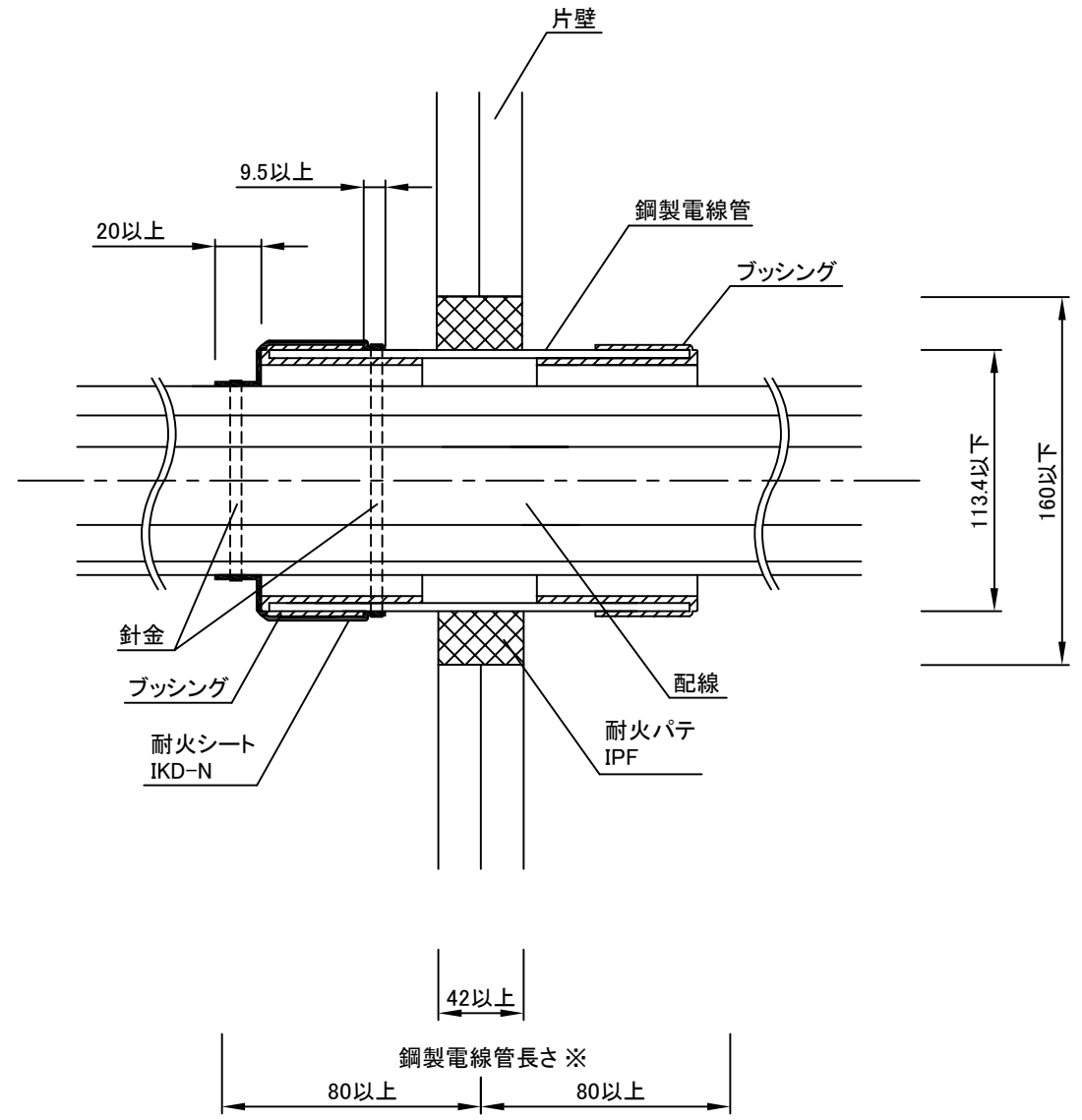
断面図
