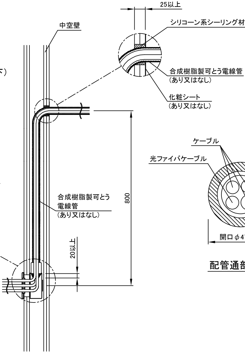
断面図
