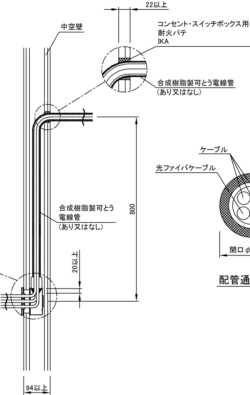
断面図(壁内部)
