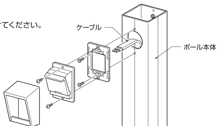
【EV充電コンセント施工例】
