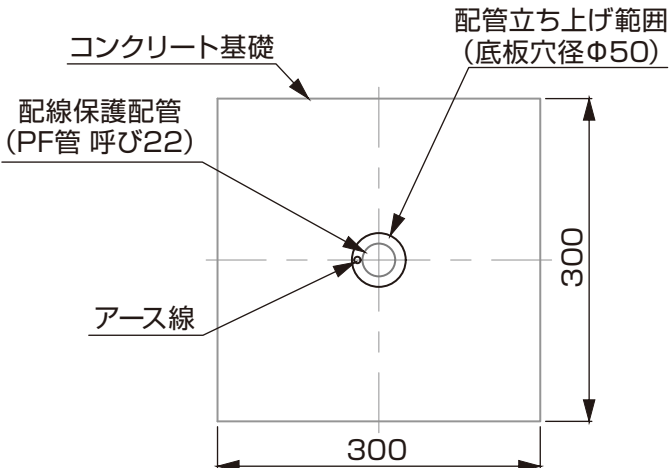
上面図／配管立ち上げ範囲（埋込配管の場合）
