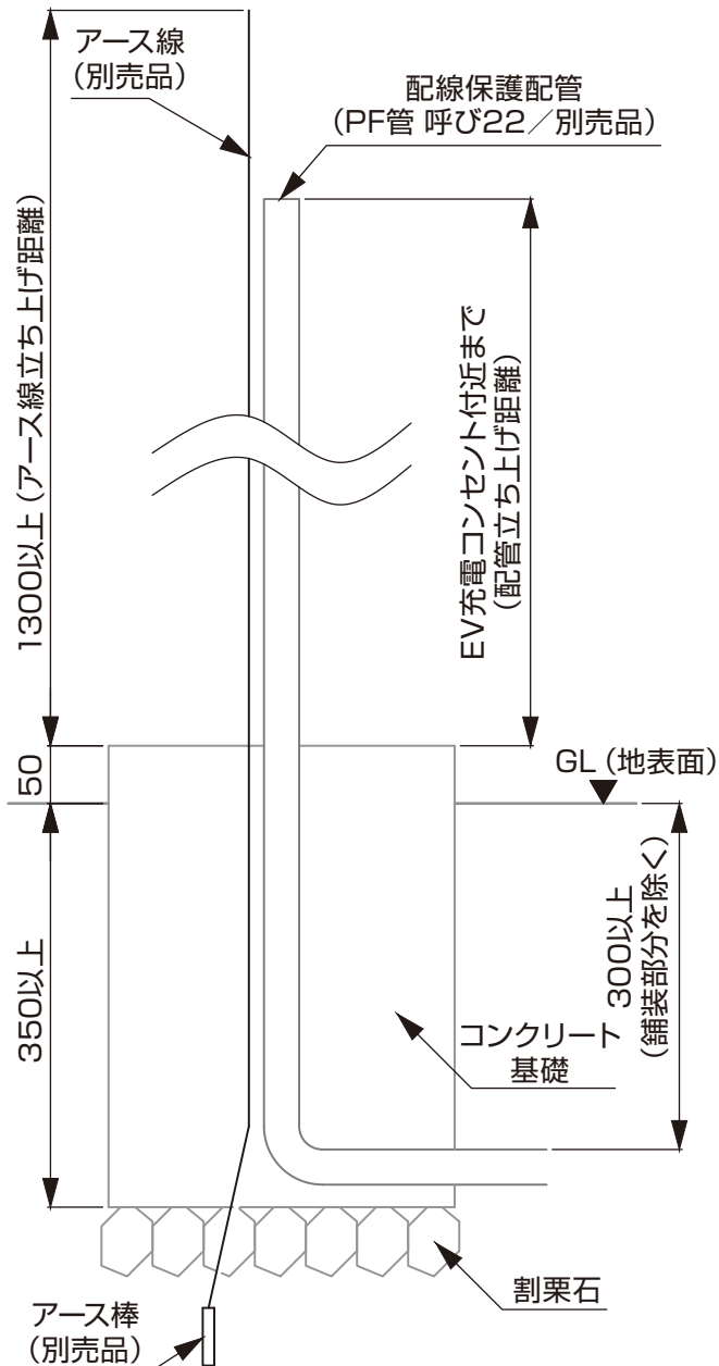
側面図／配管深さ・立ち上げ（埋込配管の場合）
