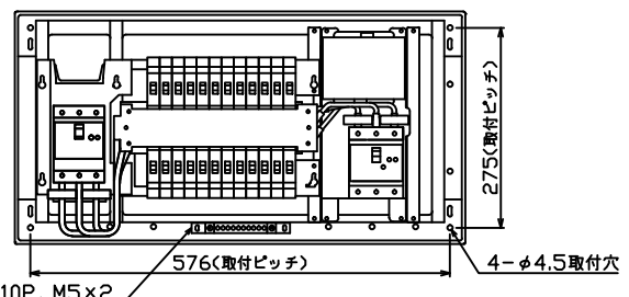
連結式7-ス中継端子 10P, M5×2
