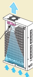
静音冷却ファン
